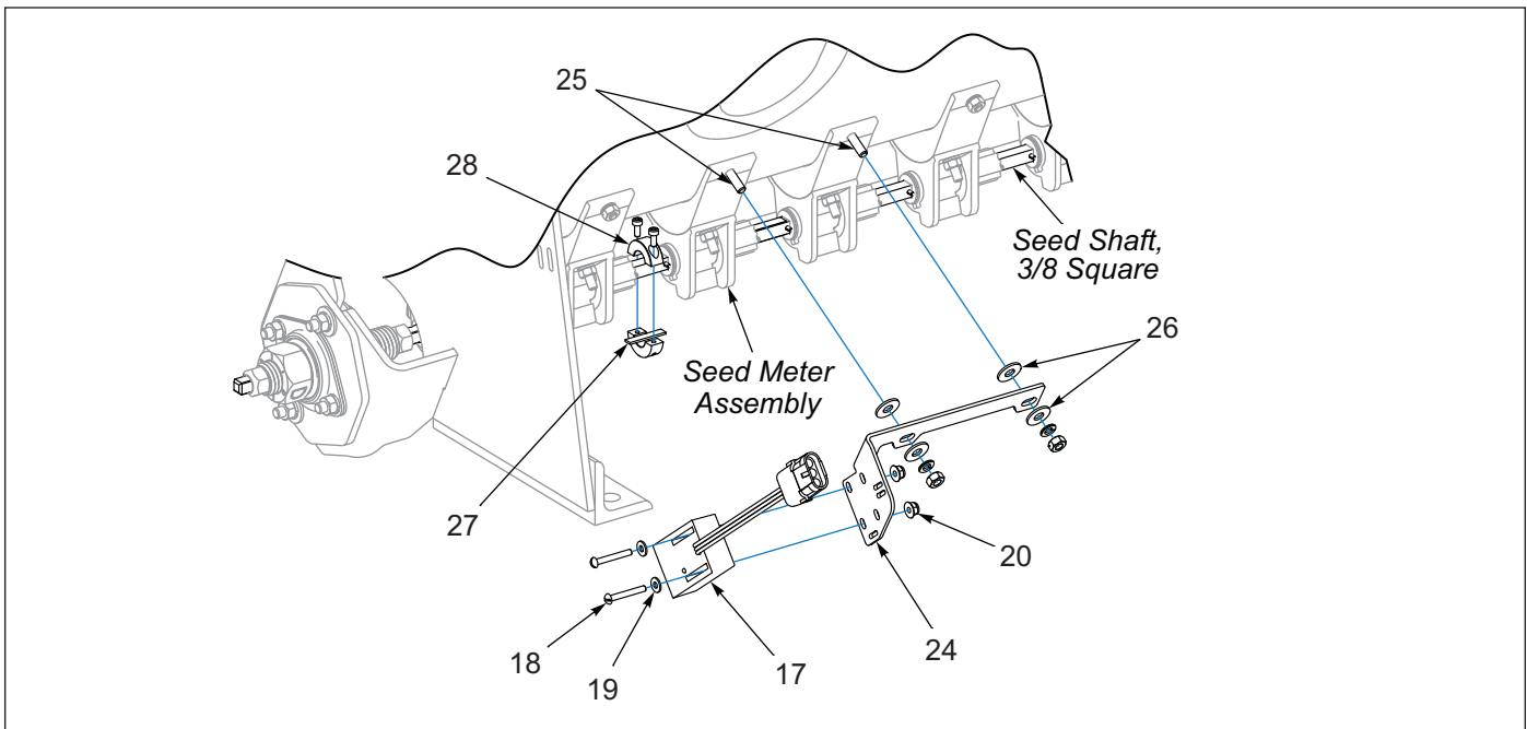
Figure 1-53: Brillion Elite Mini Monitor - Seed Shaft Sensor
