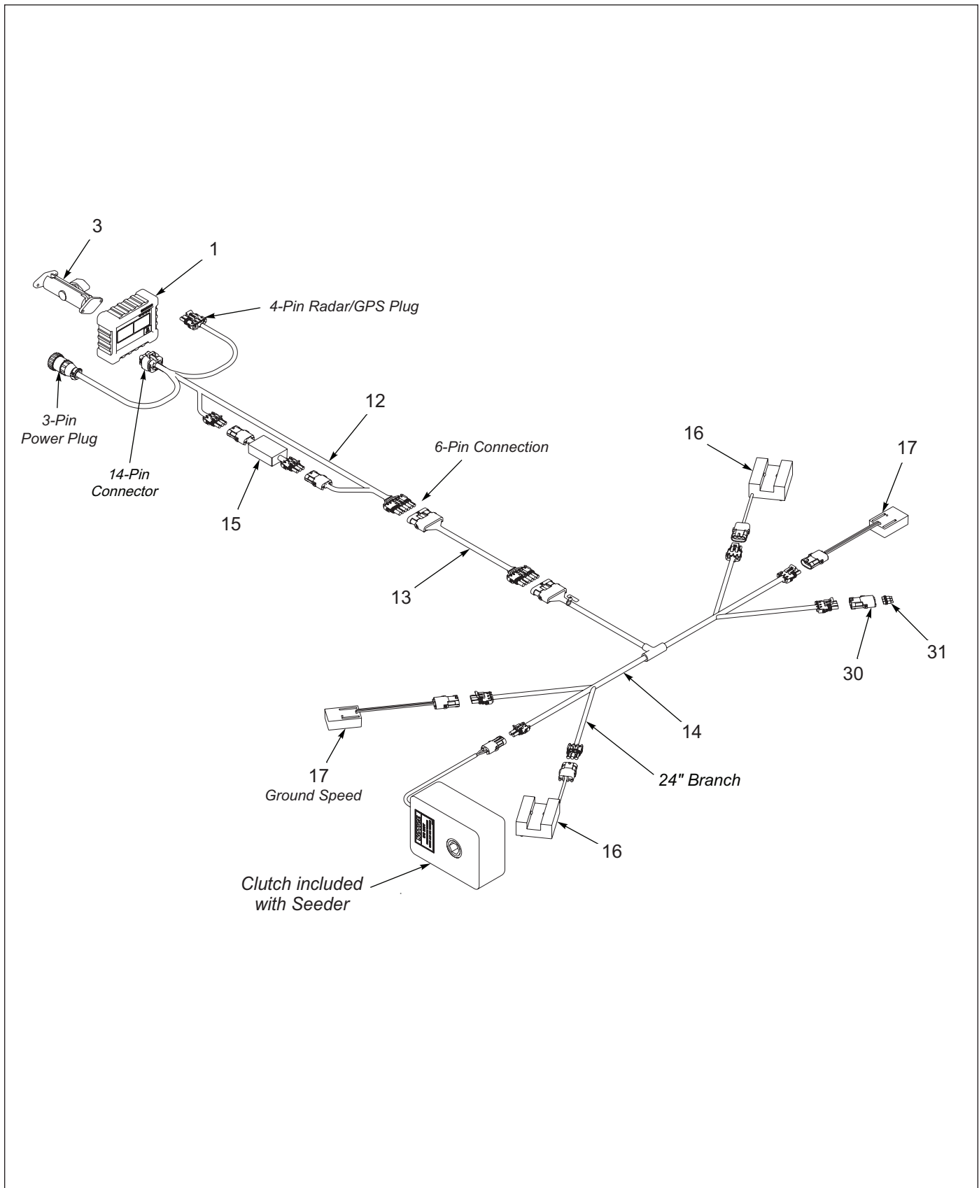
Figure 1-53: Brillion Elite Mini Monitor Electrical Schematic
