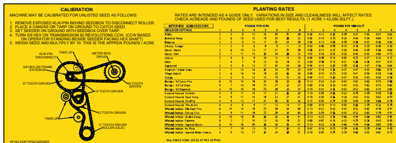
ITEM 8 - 2P104
